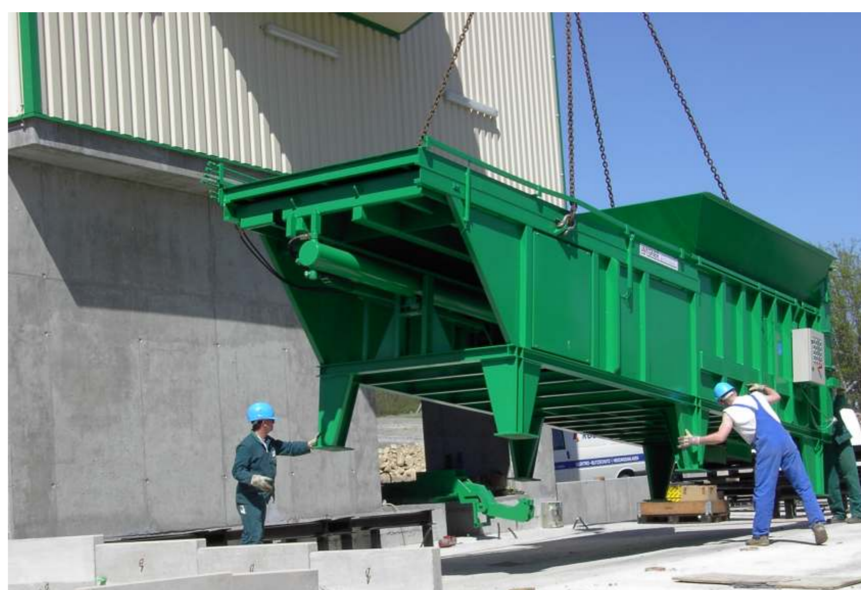
Mai 2003: Einbau der Presse, 14.200 kg Gewicht, 8,1 m x 2,4 m x 3,6 m (L x B x H)
